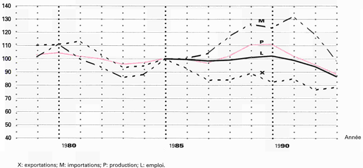
Secteur de la construction de machines et de matériel mécanique de l'EUR 12: production, emploi, importations et exportations. 1985 = 100
