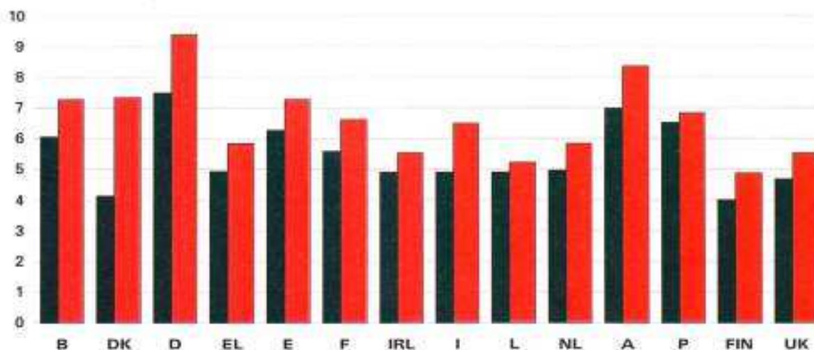
Prix de l'électricité pour gros usagers industriels types; 24 GWh par an, en ECU par 100 kWh, 1 er juillet 1995
